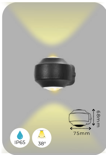
12W Platio 6X2
